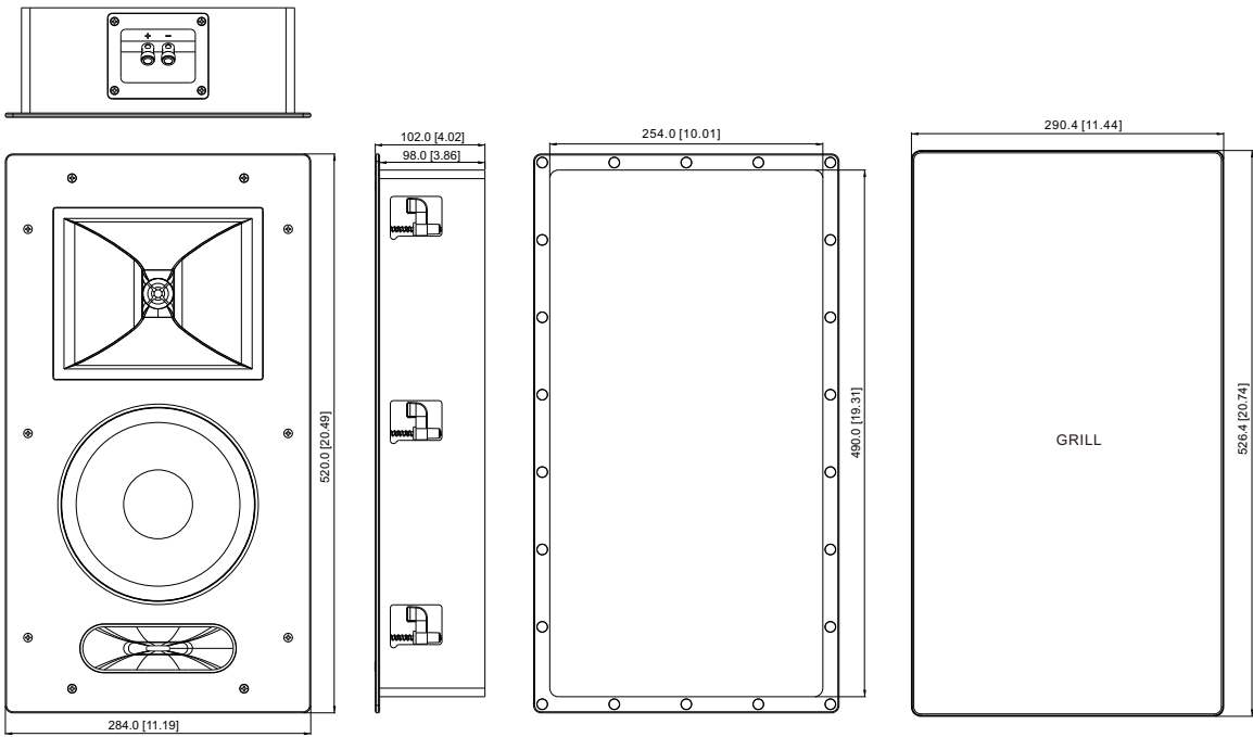
X8成品尺寸
