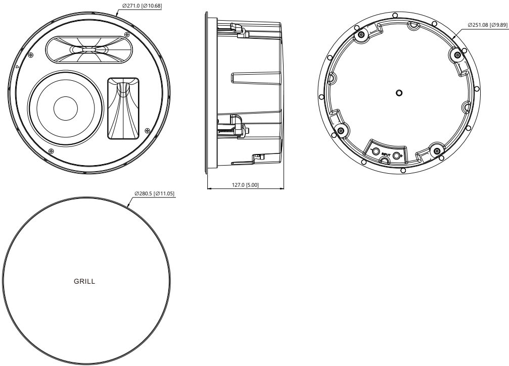
X6成品尺寸
