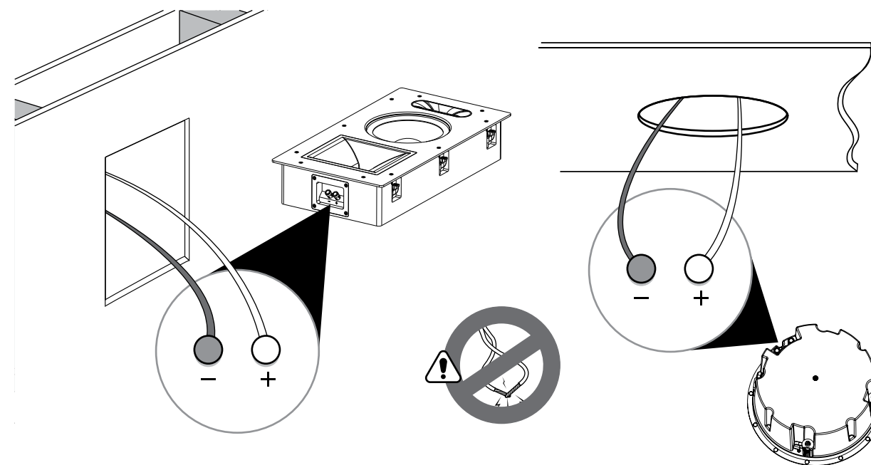
③ 开孔后将音箱线从孔内穿出与音箱连接（注意正负极）
